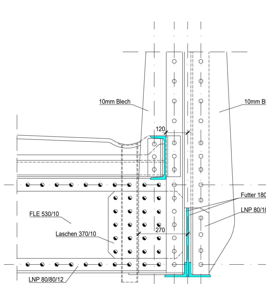
Schnitt B-B 1:10
