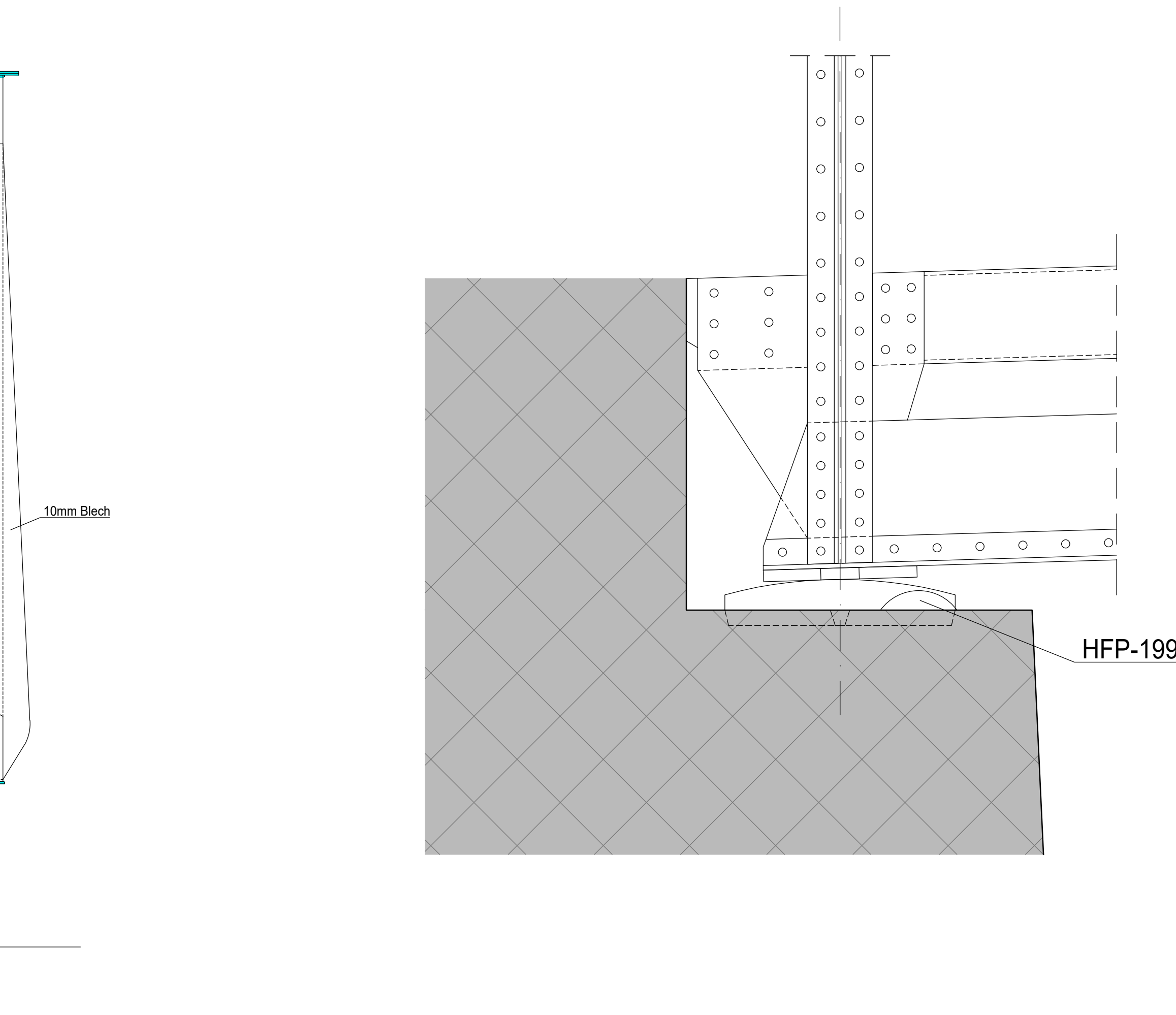
Detail Vermessungspunkt HFP-199 1:10
