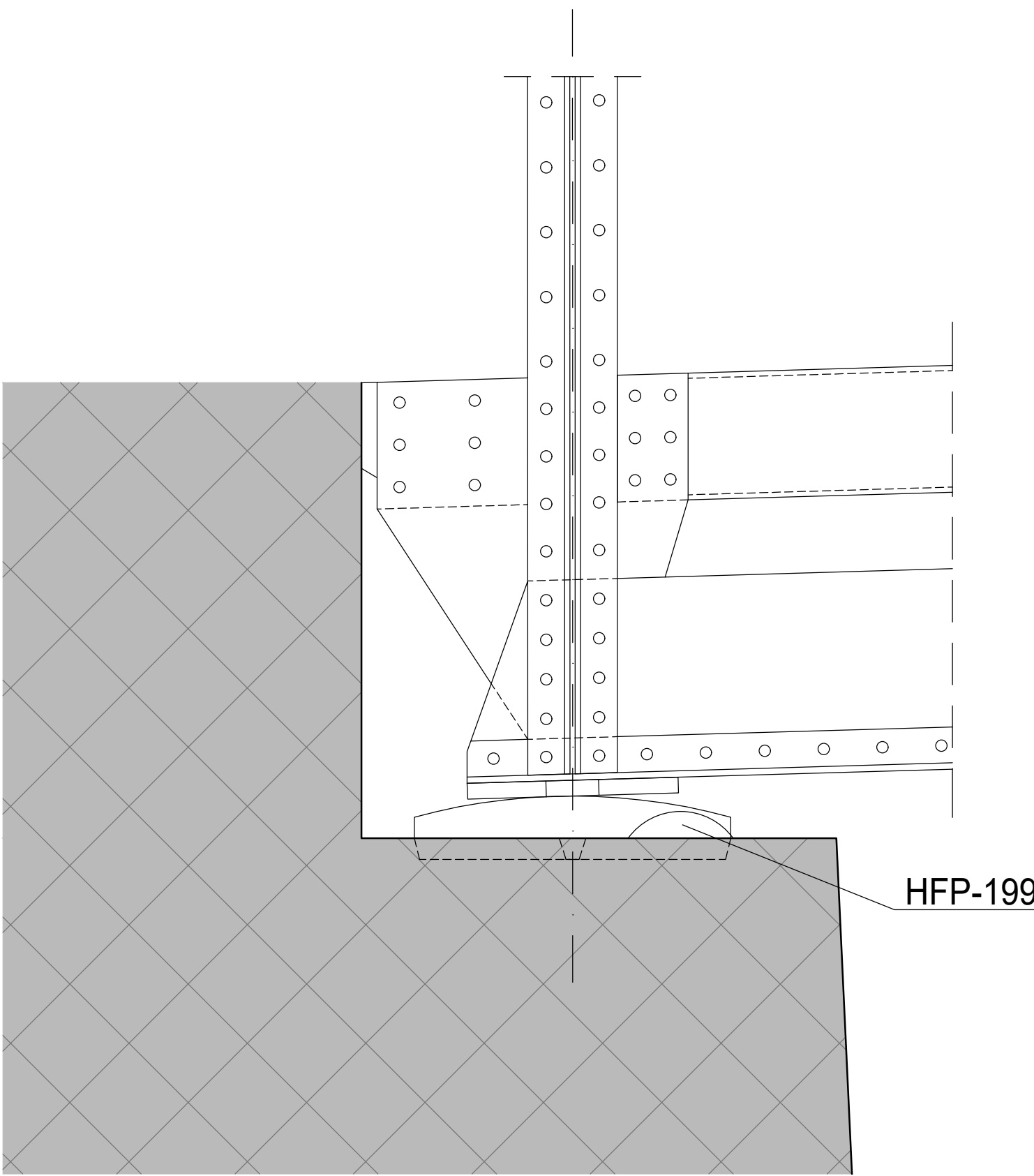
Detail Vermessungspunkt HFP-199 1:10
