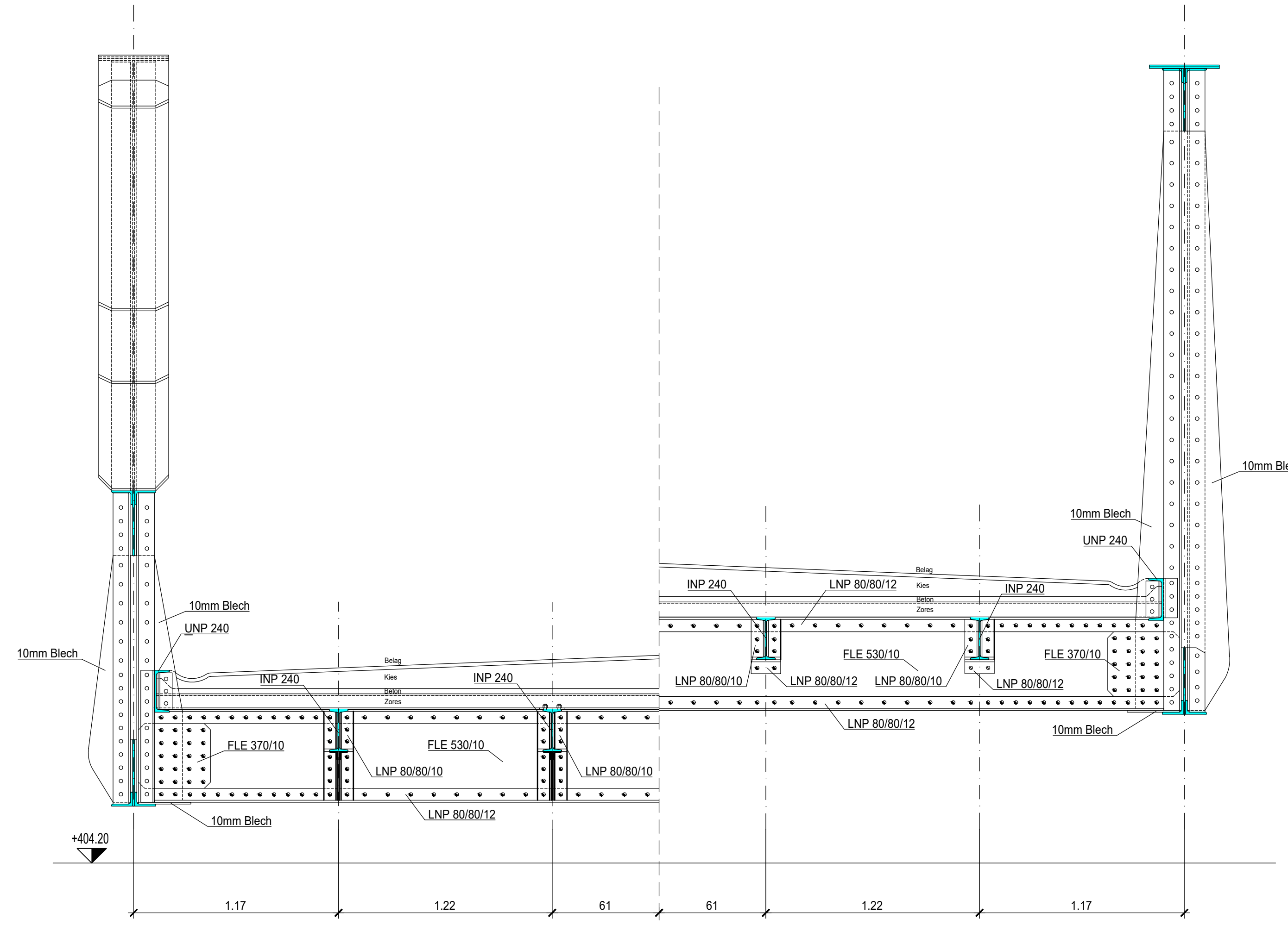
Querschnitt D-D 1:20
