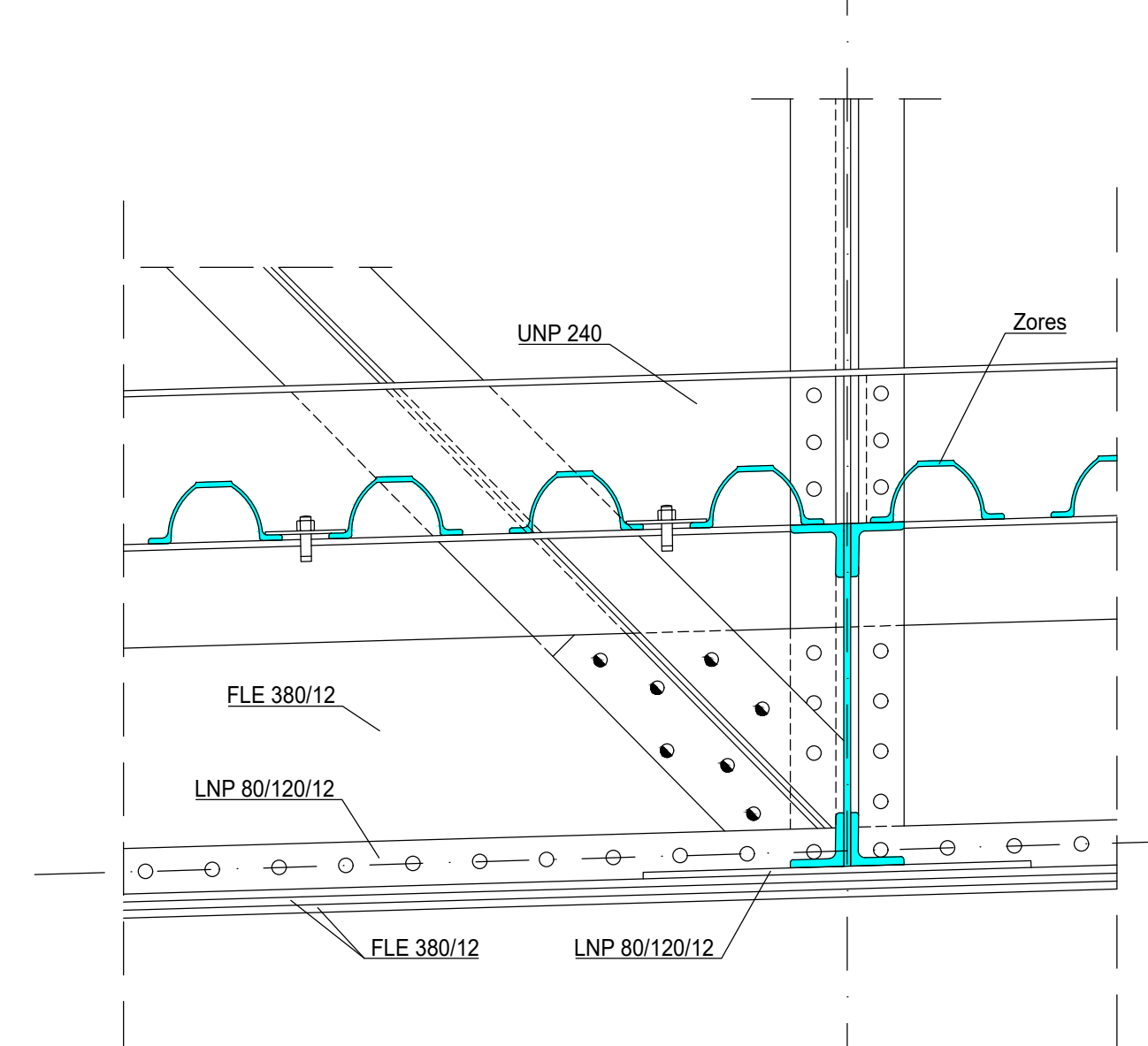
Schnitt A-A 1:10
