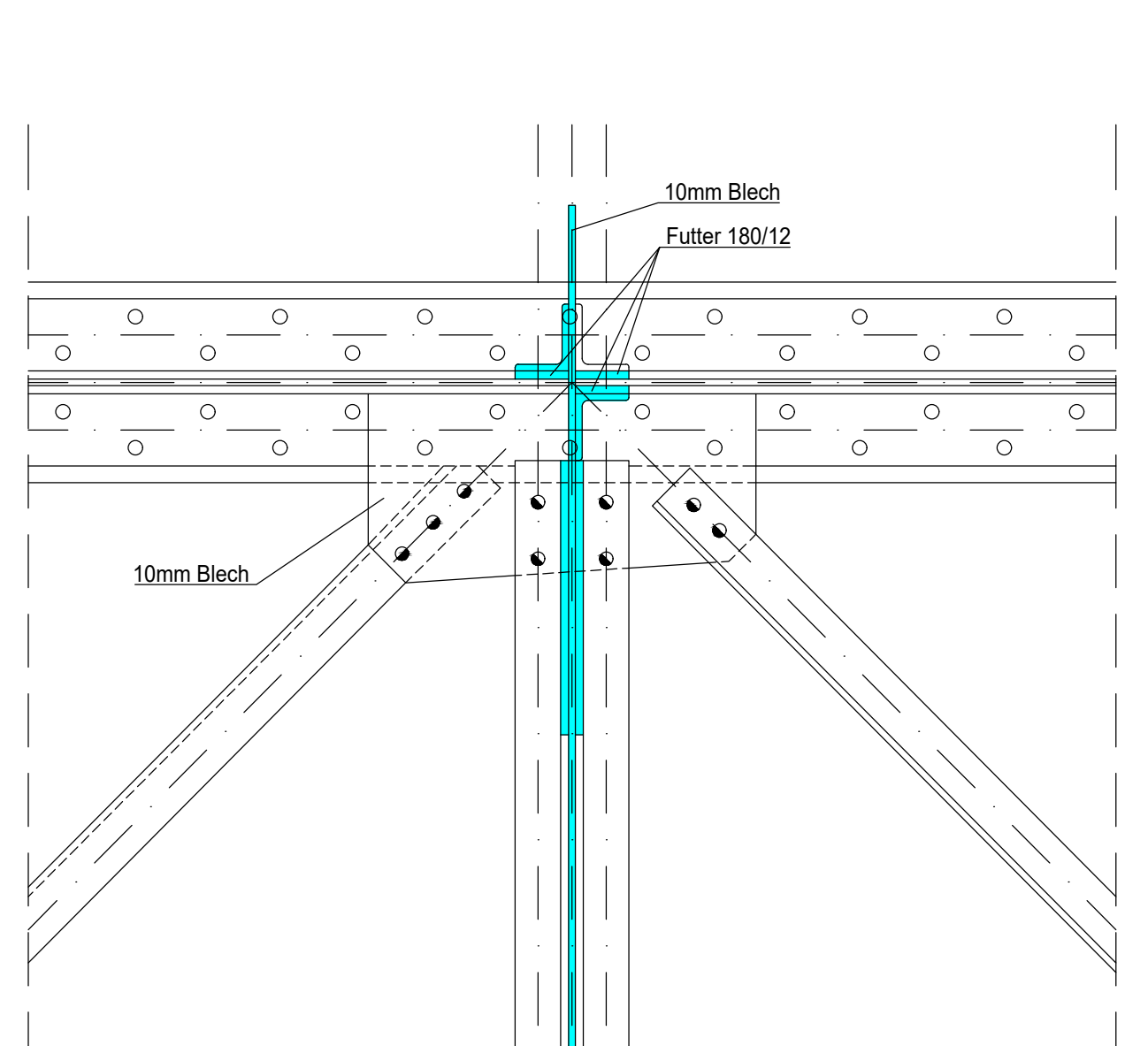
Schnitt C-C 1:10
