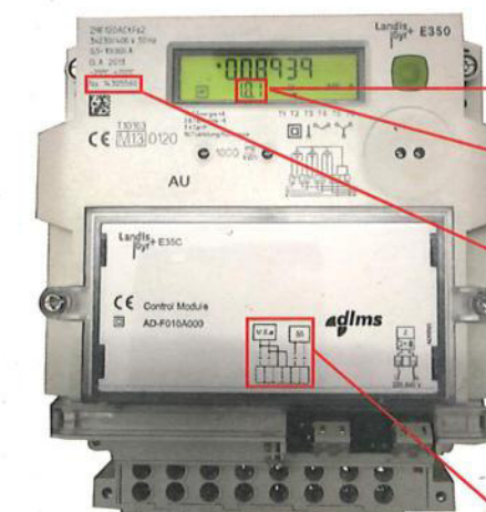
Smartmeter Landis+Gyr E350
