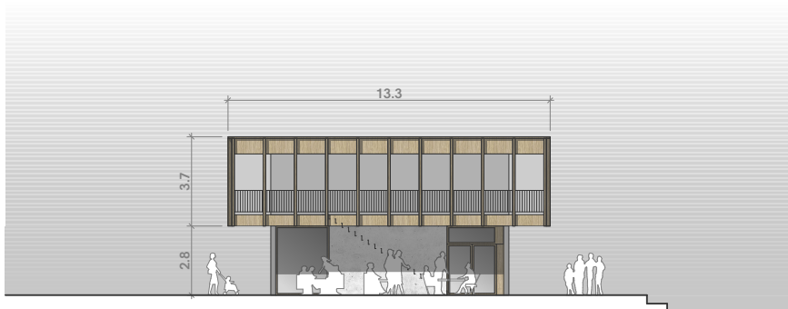
Südansicht
